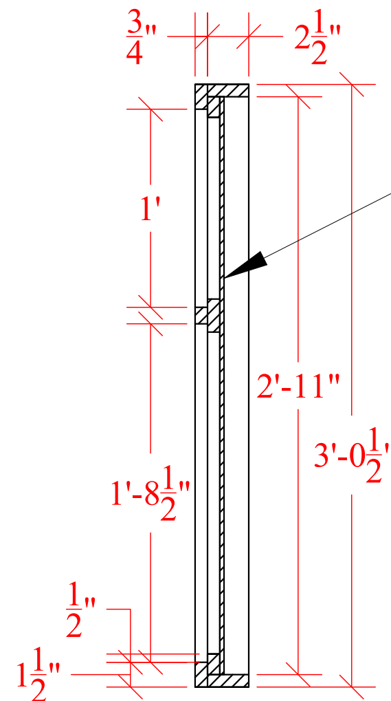
SECTION A-A
